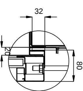
DETTAGLIO 5 SCALA 1:4
