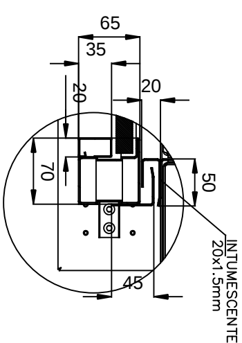
DETTAGLIO 3 SCALA 1:4
