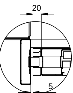
DETTAGLIO 4 SCALA 1:4
