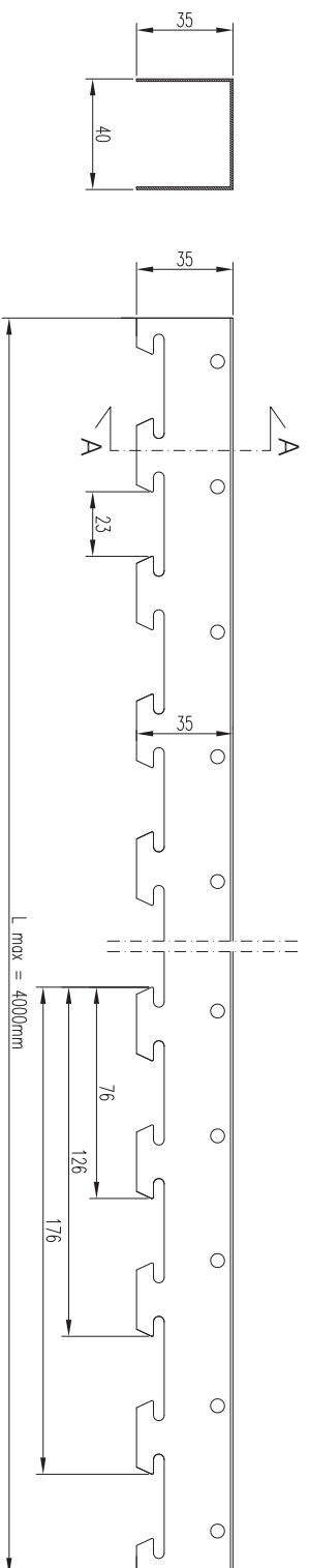
A-A SECTION
