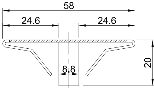
A-A SECTION
