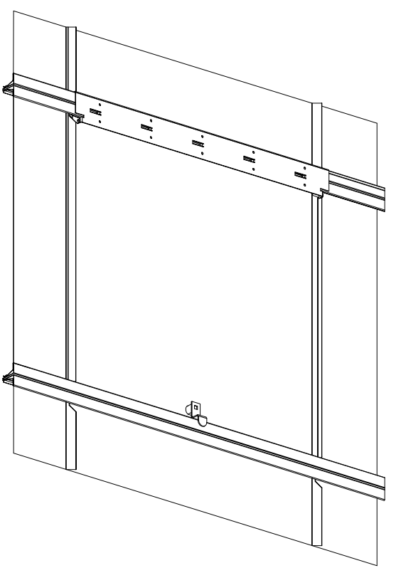
ASSONOMETRY
