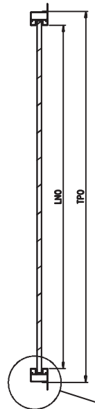
SEZIONE B-B
